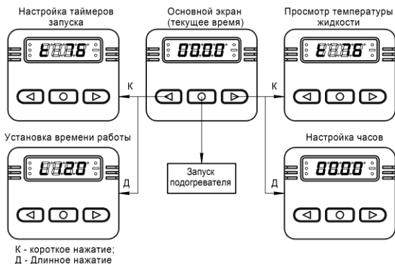
Рис. 4.2 – Алгоритм работы пульта ПУ-11 для 14ТС-10.
