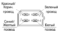
Рис. 5.1 – Установка контактов в колодку.
