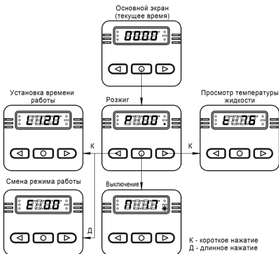
Рис.4.9 – Запуск подогревателя 14ТС-Mini в режиме «предпусковой»
