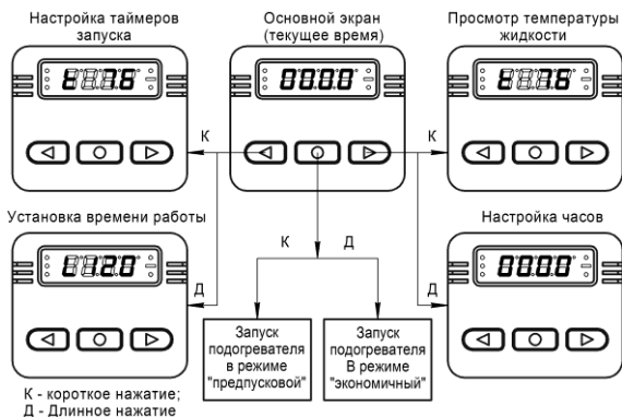
Рис. 4.3 – Алгоритм работы пульта ПУ-11М для 14ТС-Mini.
