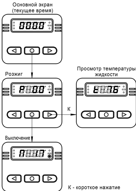
Рис.4.8 – Запуск подогревателя 14ТС-10
