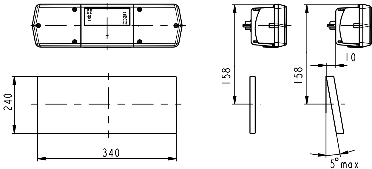
Посадочное место на автомобиле.
