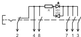
Электрическая схема/Electrical diagram
