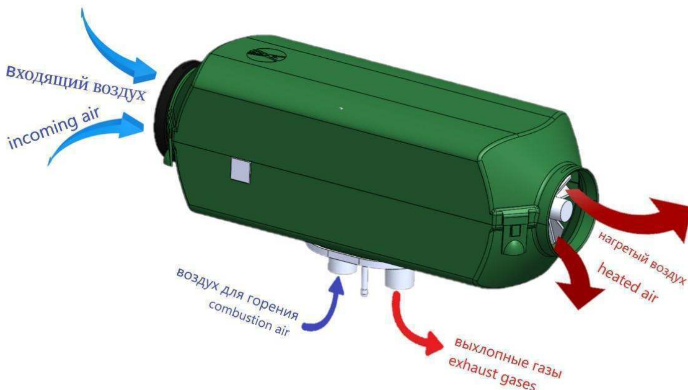
Рис.1 Нагреватель
