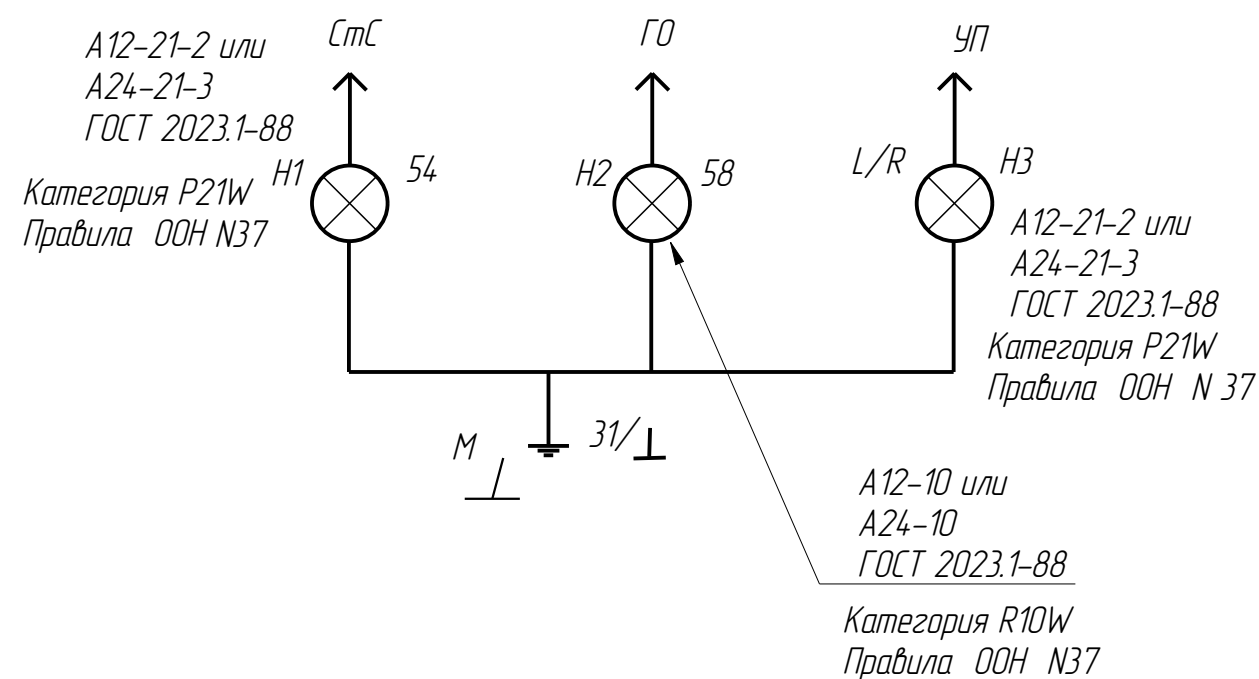
Схема электрическая принципиальная
