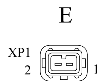
Расположение контактов на блоке управления со стороны штырей
