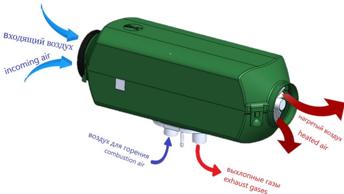
Рис.1 Нагреватель
