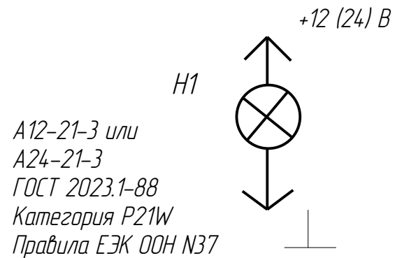
Схема электрическая принципиальная
