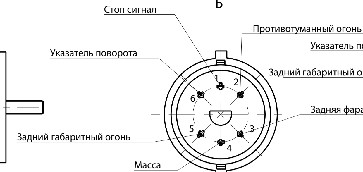
Рис.2 Вилка СЦА3-2-6-В-01
