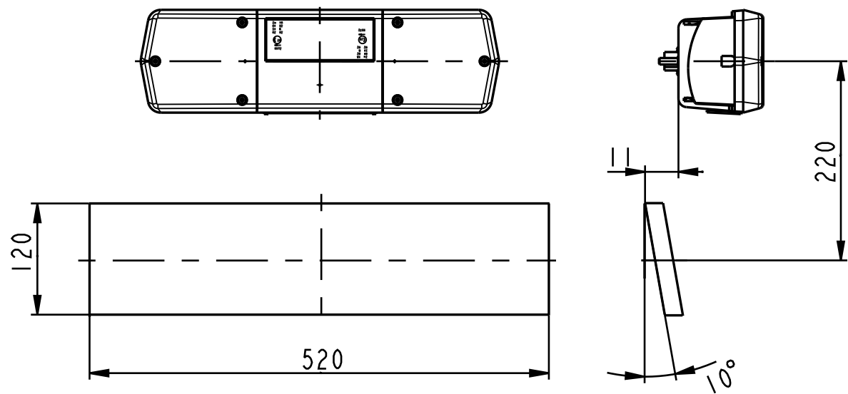
Схема установки заднего номерного знака (вариант2).
