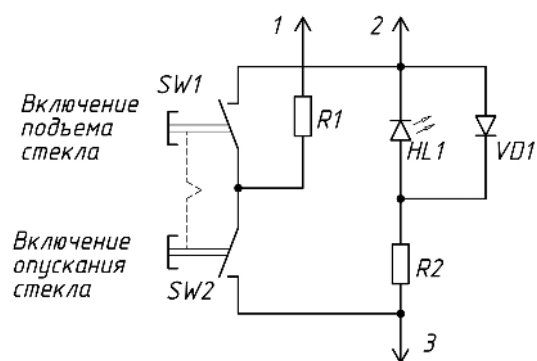
Электрическая схема/Electrical diagram
