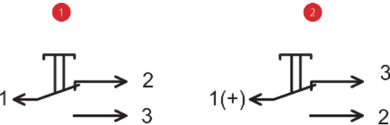
Электрическая схема/Electrical diagram
