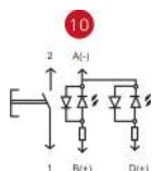
Электрическая схема/Electrical diagram
