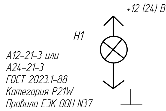
Схема электрическая принципиальная
