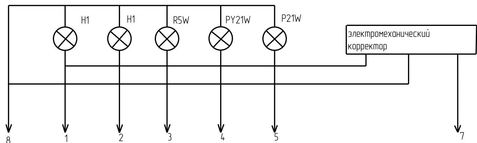
Схема электрическая
