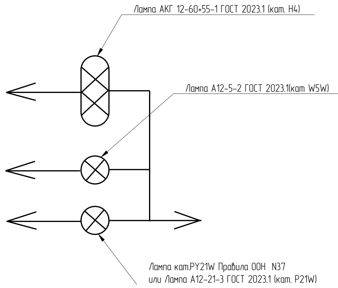
Схема электрическая
