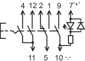
Электрическая схема/Electrical diagram
