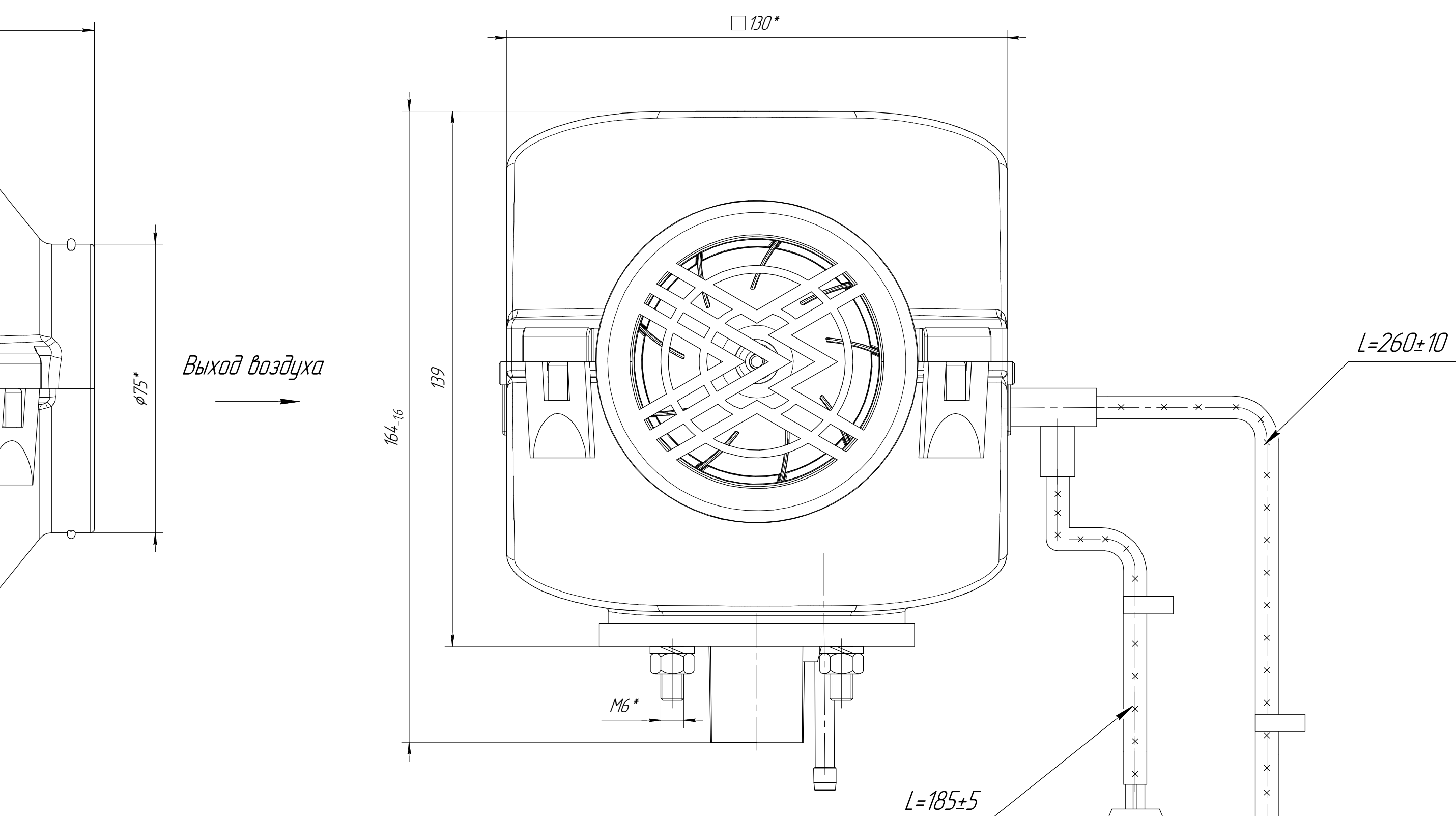
вид А
