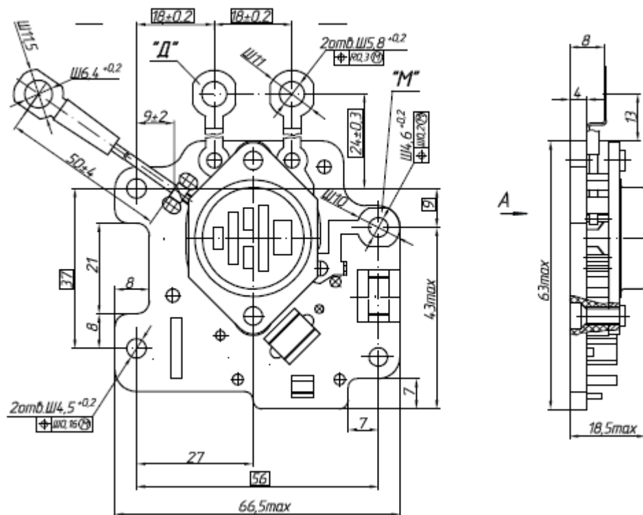
Габаритный чертеж 7901.3702А3 в устройстве регулирующем УР-1
