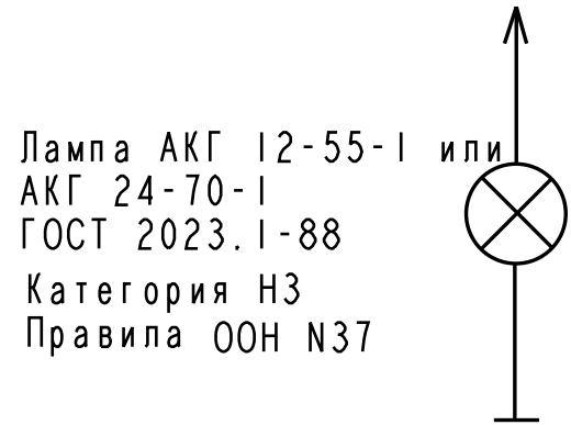
Схема электрическая принципиальная
