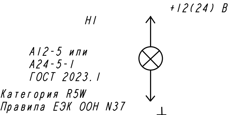
Схема электрическая принципиальная
