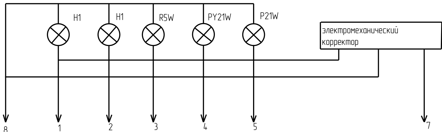
Схема электрическая
