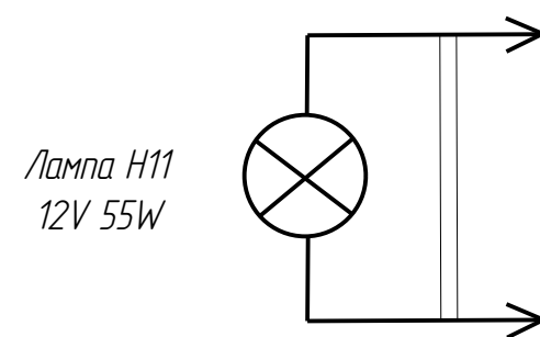
Схема электрическая
