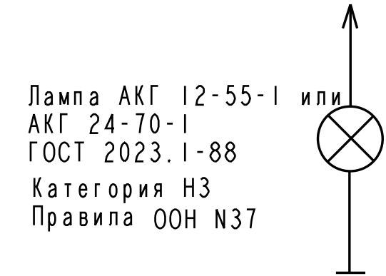
Схема электрическая принципиальная
