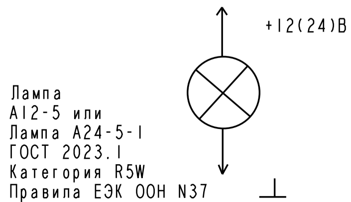
Схема электрическая принципиальная
