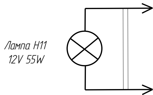
Схема электрическая
