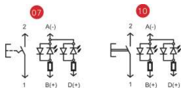
Электрическая схема/Electrical diagram
