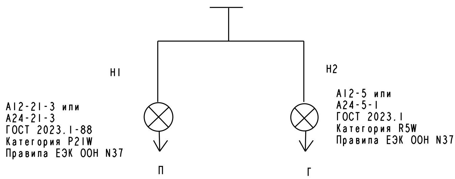
Схема электрическая
