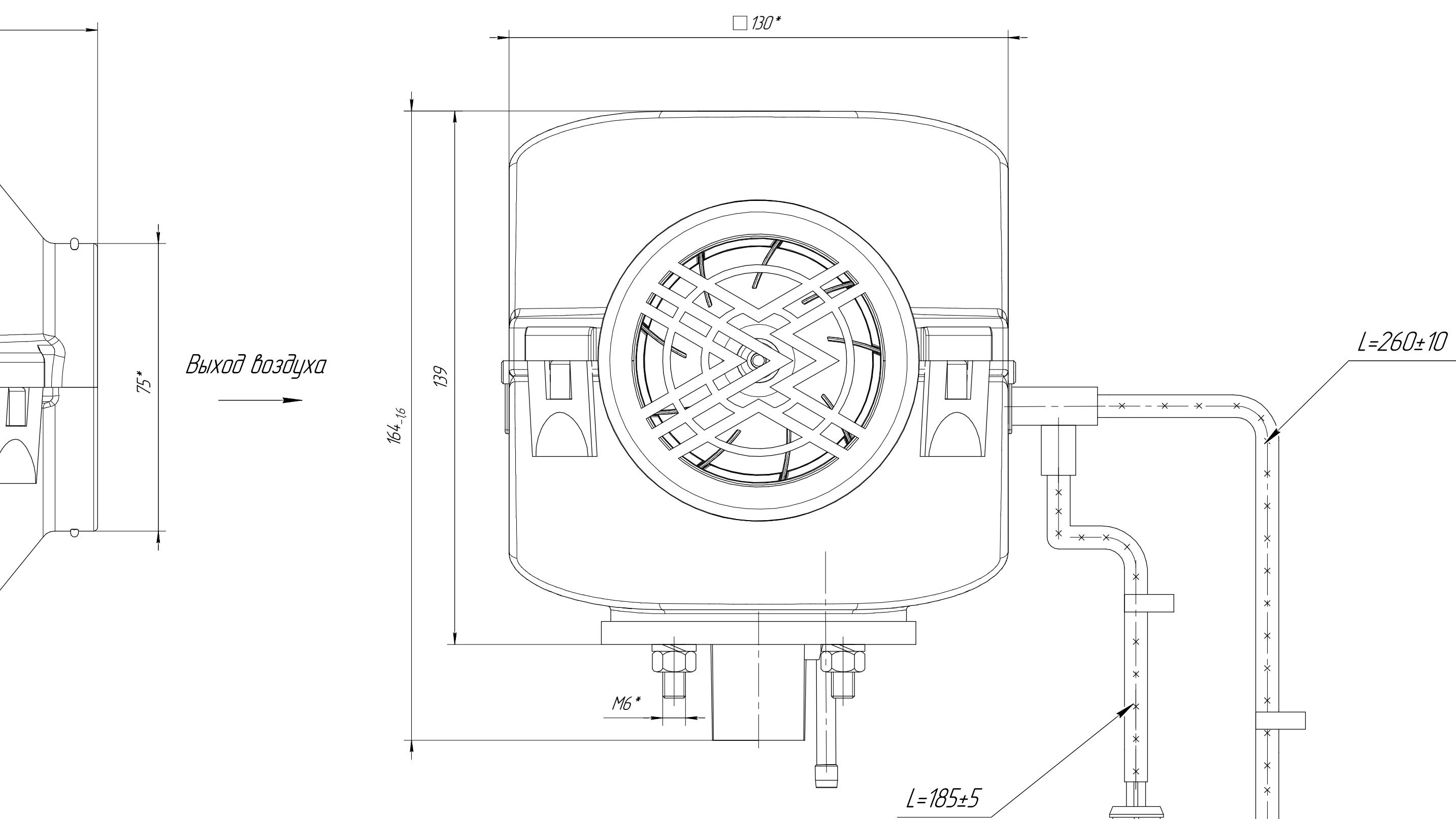
вид А
